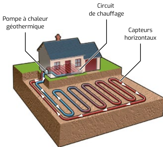
Principe d'échanges caloriques de la géothermie de surface : l'été, le bâtiment est rafraîchi par le sous-sol, plus frais que l'extérieur, et inversement l'hiver.
