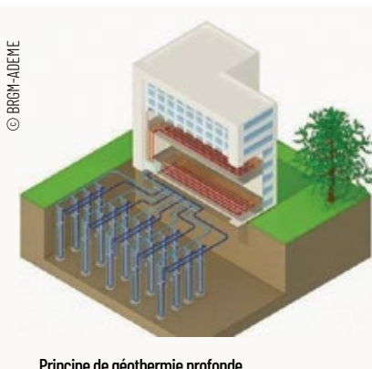
Principe de géothermie profonde.
